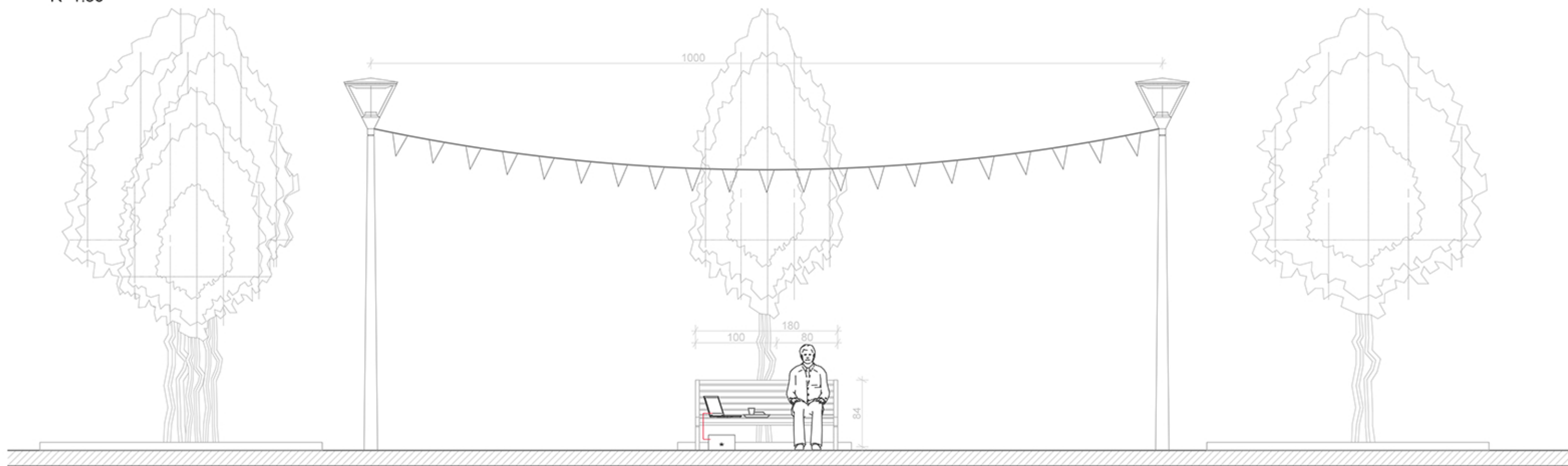
frontalni izgled E1 R 1:50
