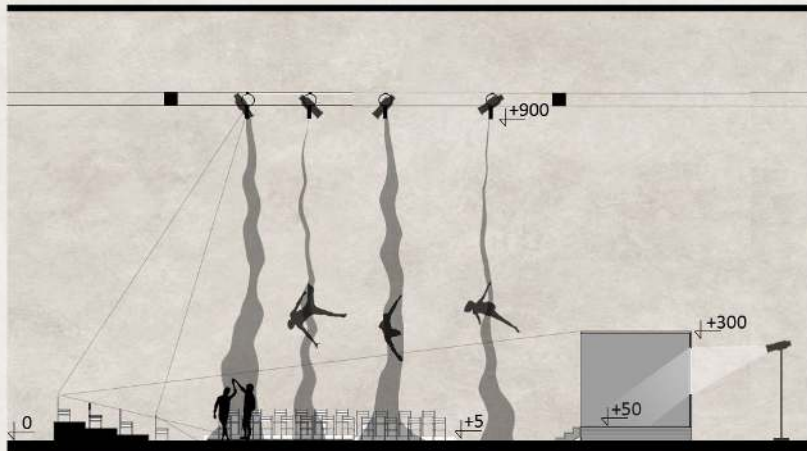
Podužni presek pozornice R=1:100
