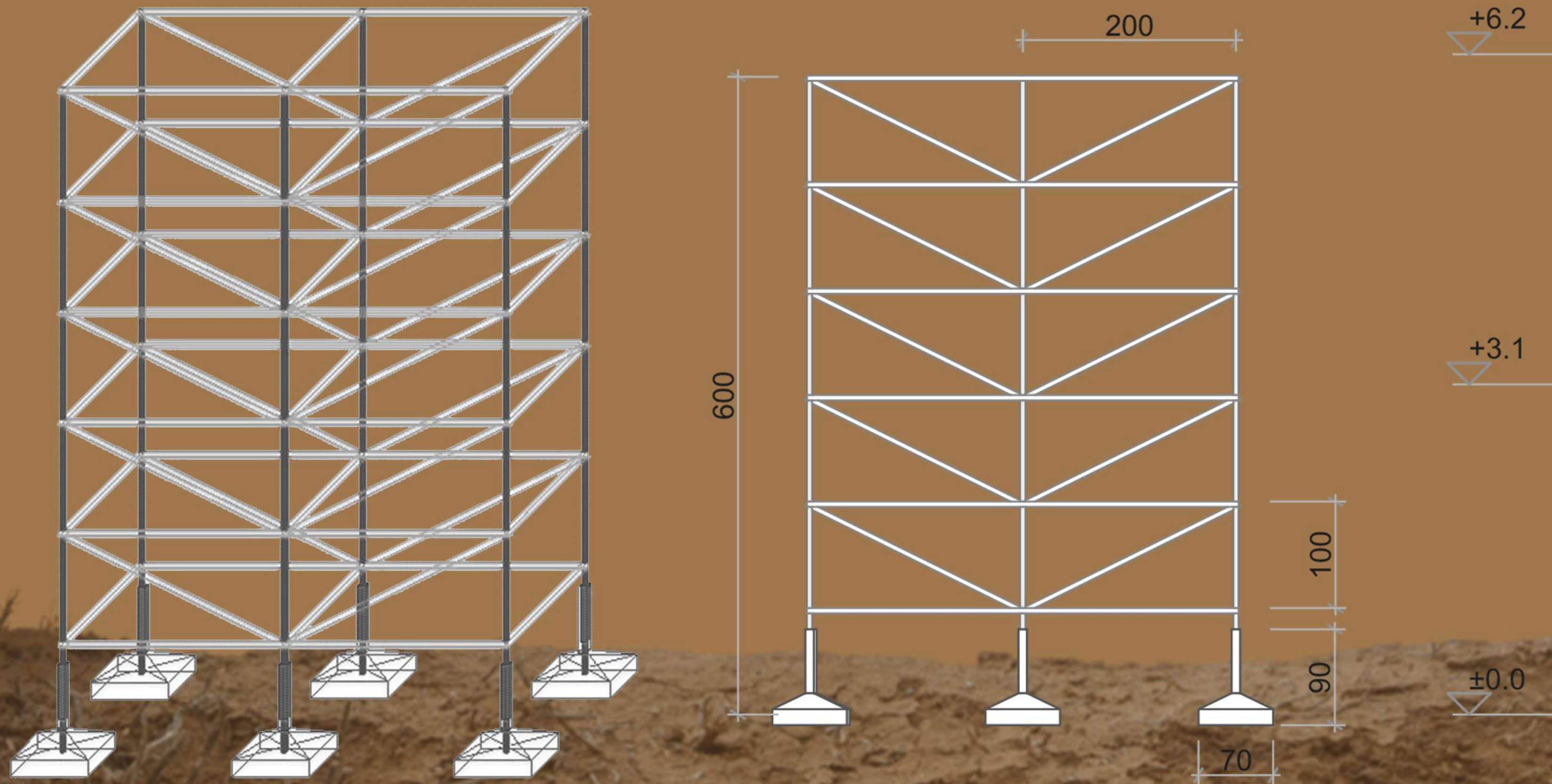
Konstrukcija skele
