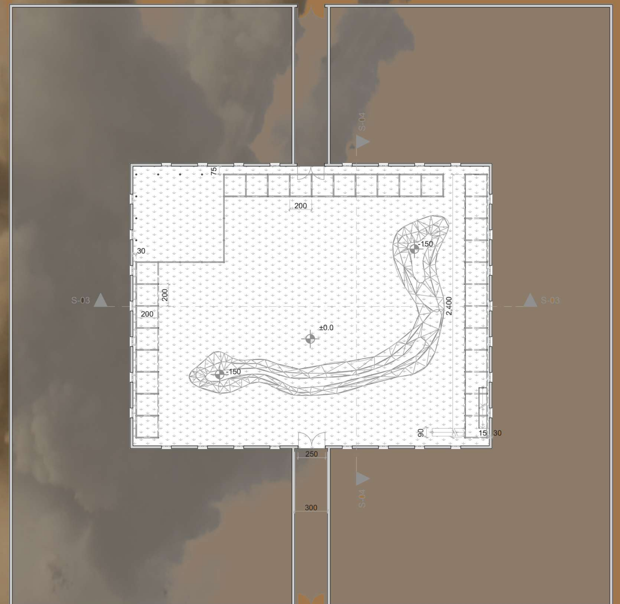
Osnova gradse kuće R 1:200
