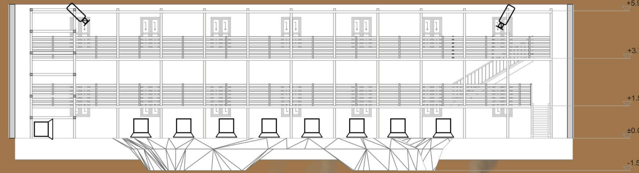
Poprečni presek atrijuma (S2) R 1:100
