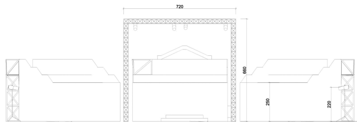
Presek C-C, 1:50
