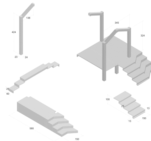
Tehničko rešenje centralne platforme
