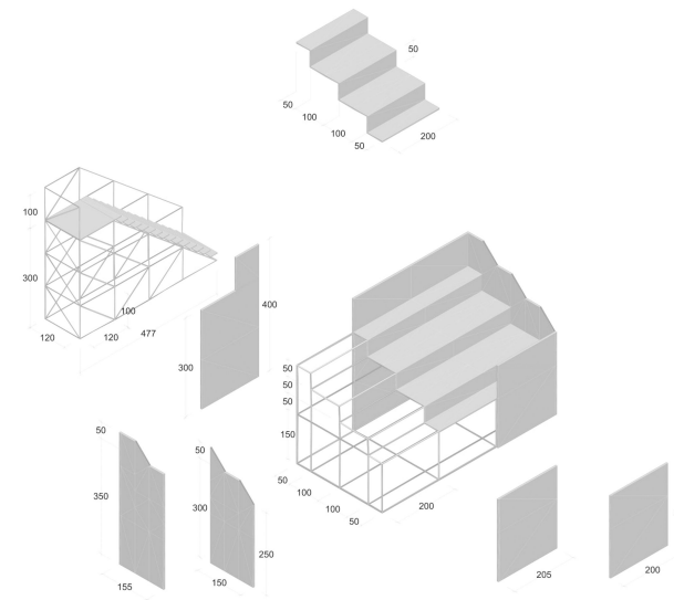
Tehničko rešenje gledališta
