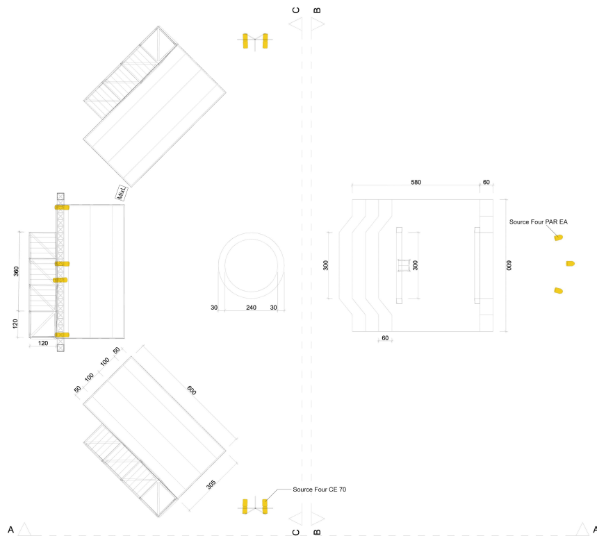
Osnova, 1:50
