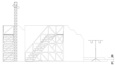
Presek A-A, 1:50
