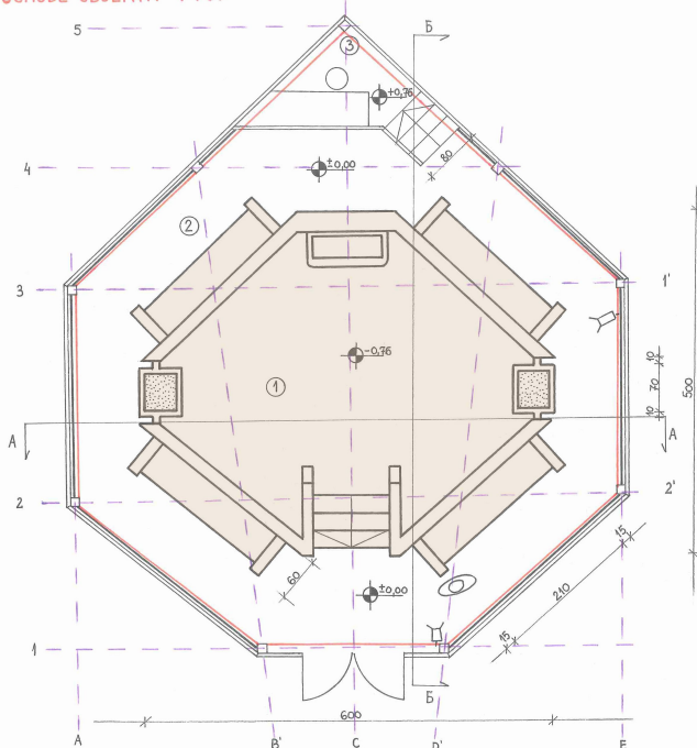
ПОЗОРИШТЕ „ПАНИКА“ ОСНОВЕ ОБЈЕКТА Р1:50
