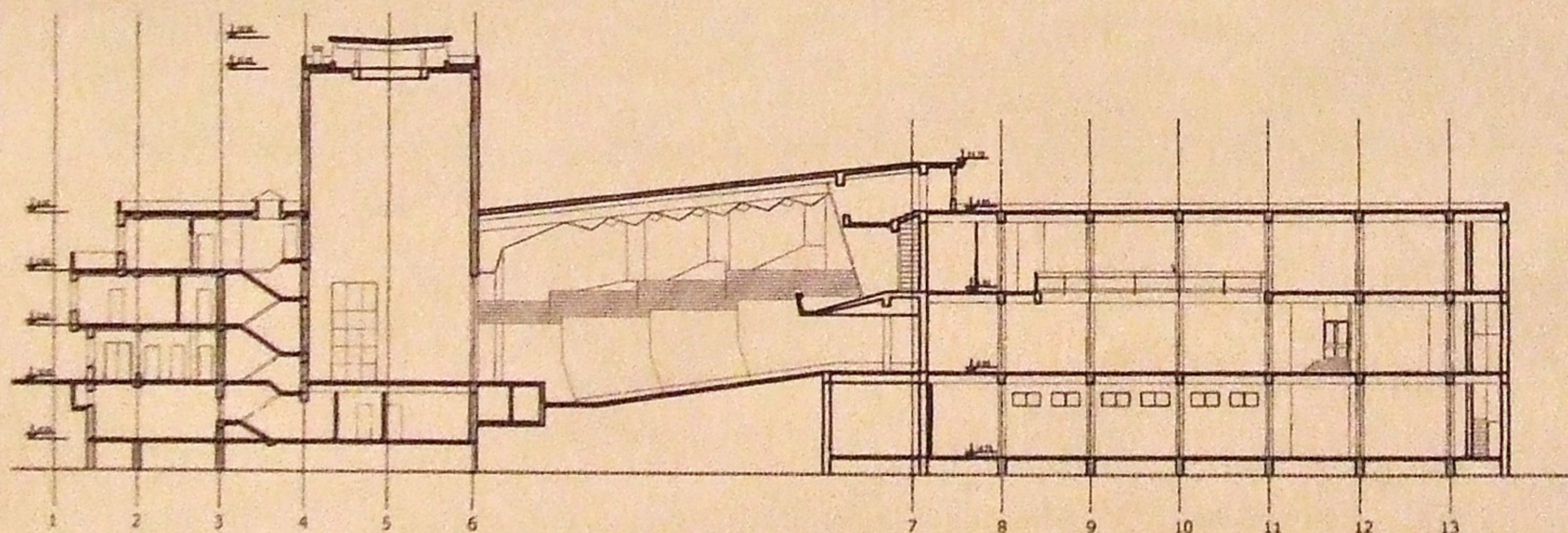
PRESEK 1-1
