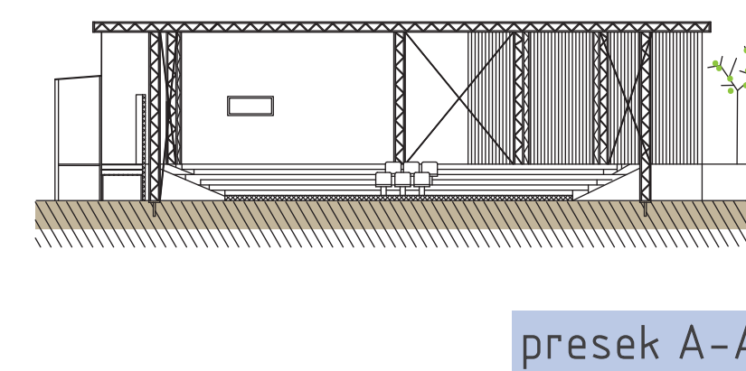
presek A-A
