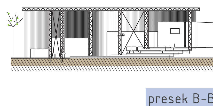
presek B-B
